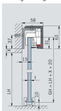
Vægmontage
