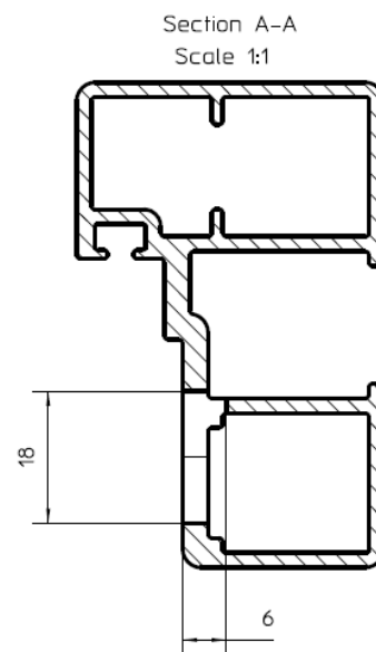
HK3101: Doorframe
